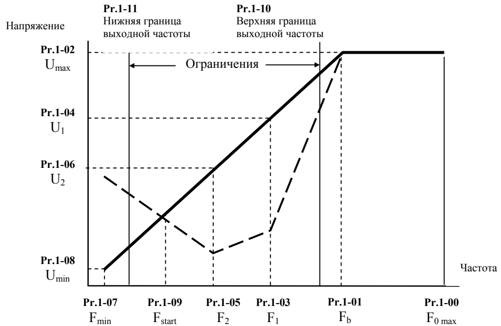
Типовая зависимость выходного напряжения от частоты U=f(F) .
